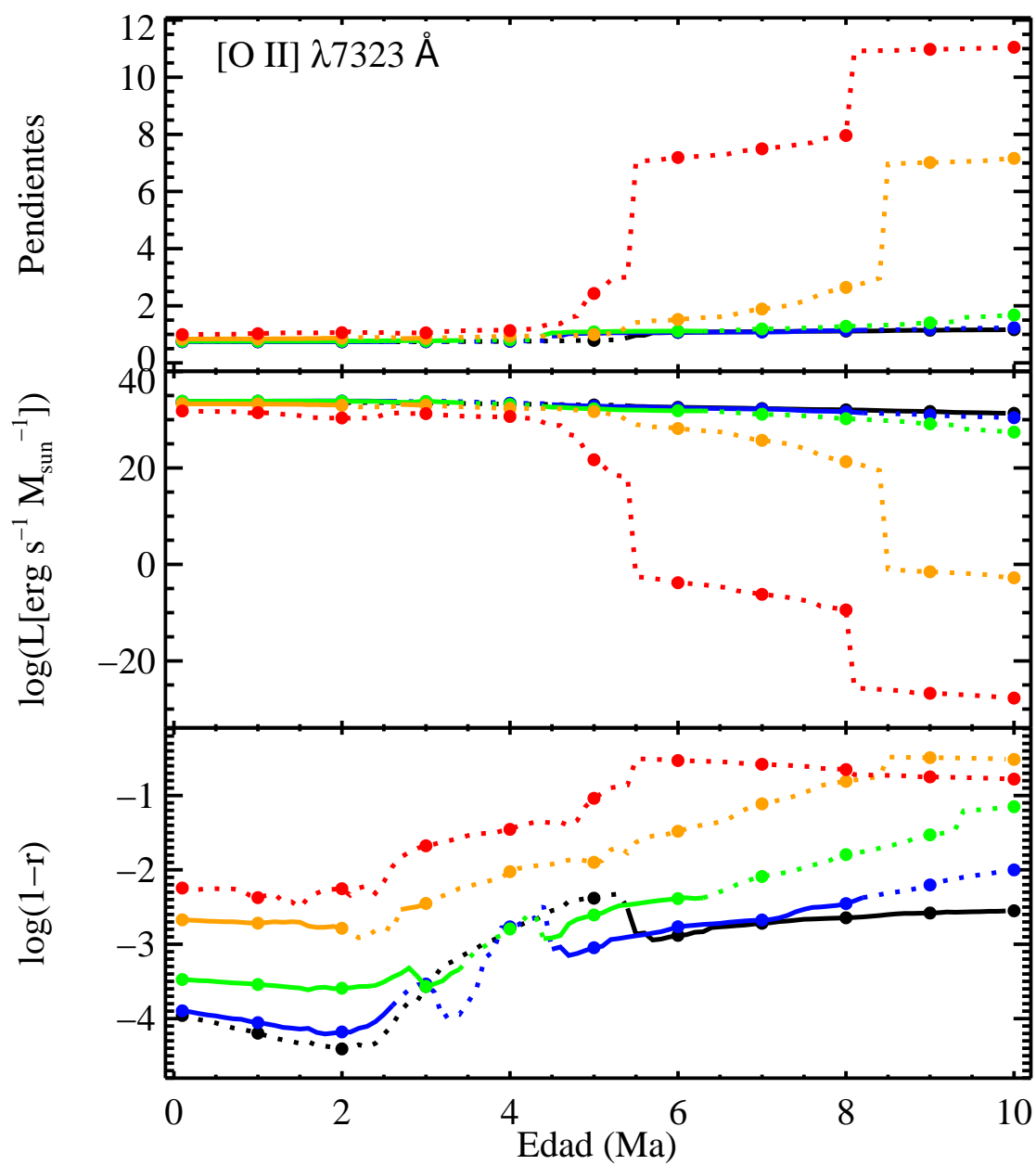
FIGURA A.23: Pendientes, \log L(1 M_{\odot}) y \log(1-r) para [O II] \lambda 7323 \text{ \AA} .
