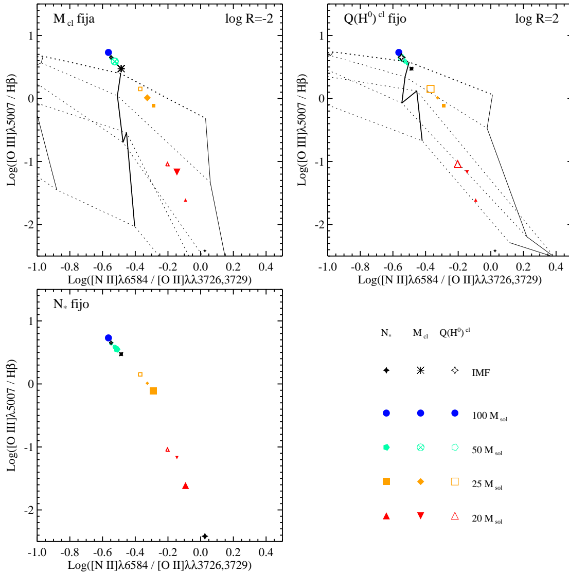
FIGURA 2.17: Diagramas de diagnóstico [\text{O III}] 5007/\text{H}\beta frente a [\text{N II}] 6584/[\text{O II}] 3726, 3729 . Símbolos como en Fig. 2.14.
