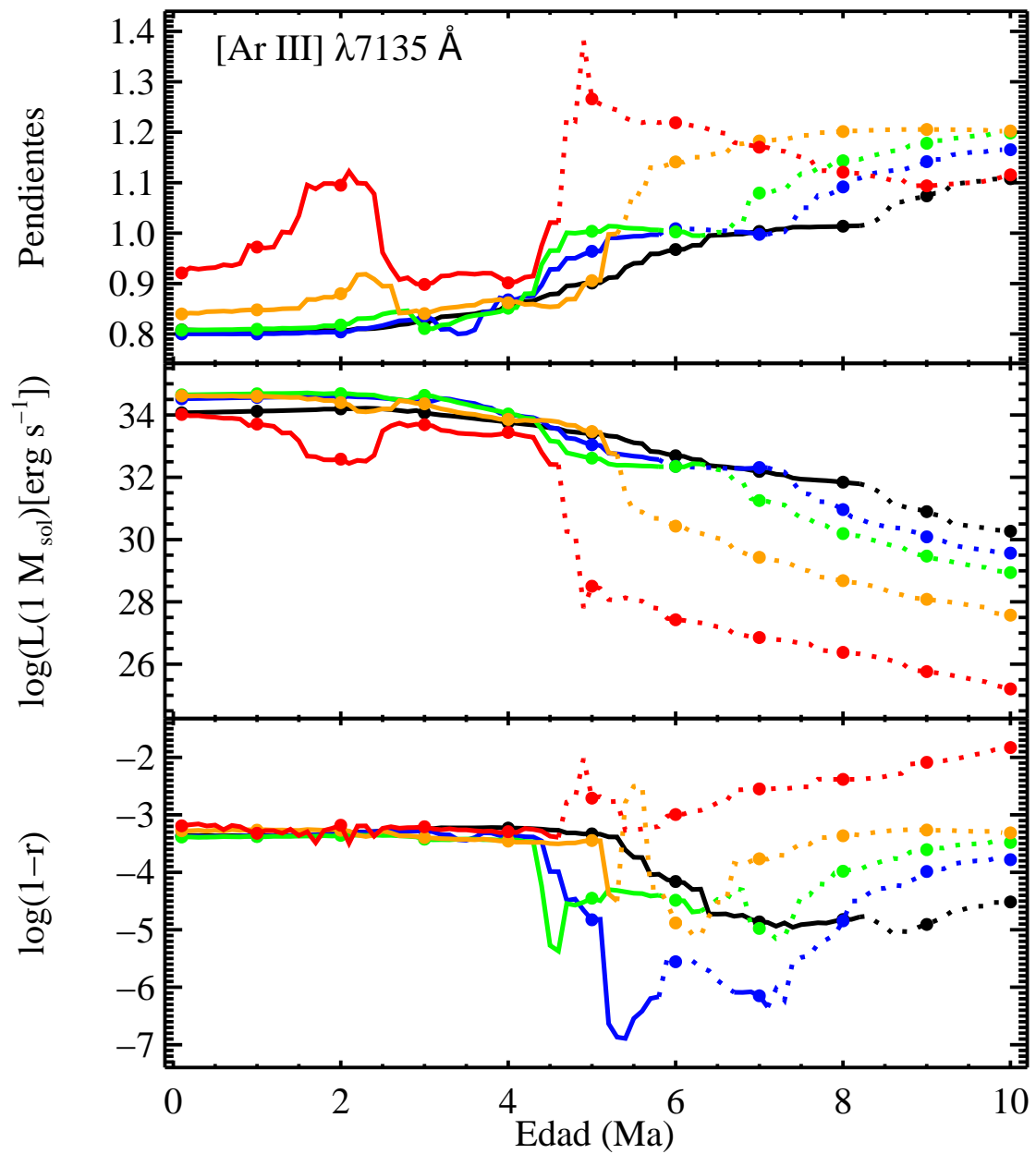
FIGURA B.22: Pendientes, \log L(1 M_{\odot}) y \log(1-r) para [Ar III] \lambda 7135 \text{ \AA} .
