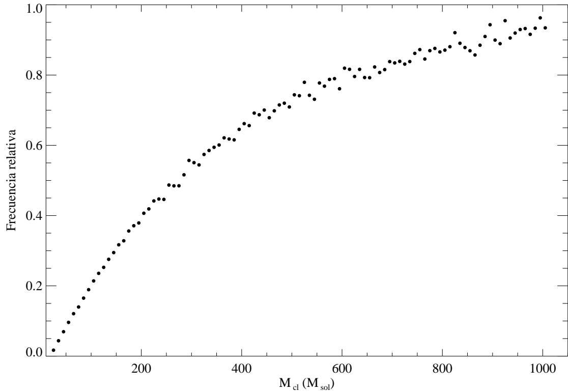
FIGURA 3.15: Frecuencia relativa de que un cúmulo tenga un continuo ionizante capaz de generar una region H II en función de su masa.
