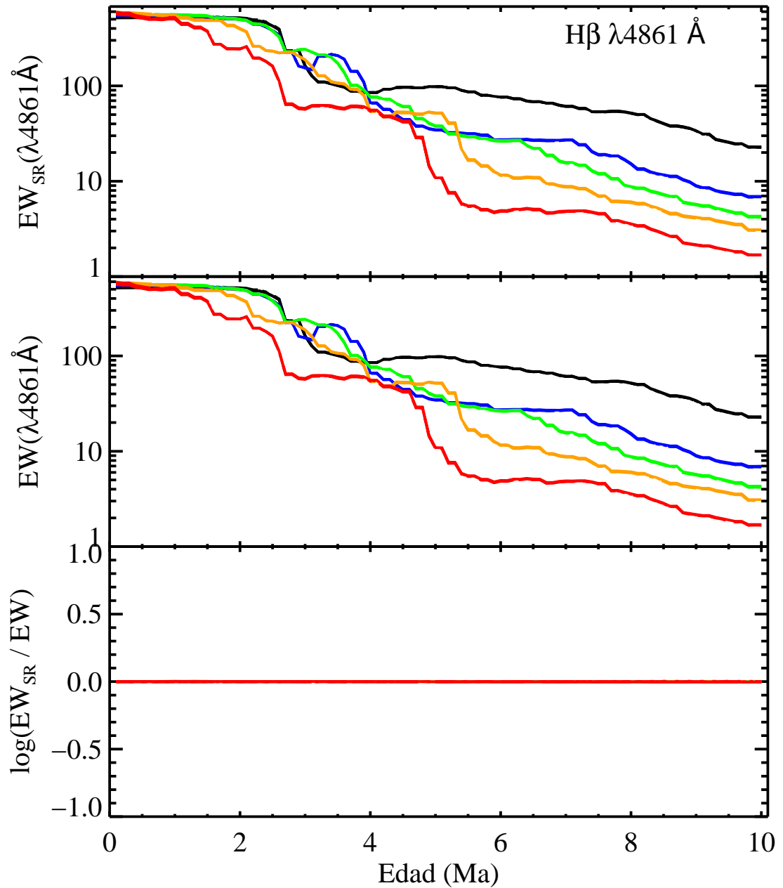
FIGURA 4.12: Anchuras equivalentes de la línea H\beta frente a la edad para M_{cl} \geq 10^3 M_{\odot} y todas las metalicidades. De arriba a abajo: Anchuras equivalentes obtenidas a partir de las relaciones de escala, anchuras equivalentes obtenidas directamente de los modelos y diferencias entre ambas. El trazo de la línea representa la masa. Raya larga: 10^3 M_{\odot} . Raya-punto: 10^4 M_{\odot} . Puntos: 10^5 M_{\odot} . Raya corta: 10^6 M_{\odot} . Continua: 10^7 M_{\odot} . Colores como en Fig. 4.1.
