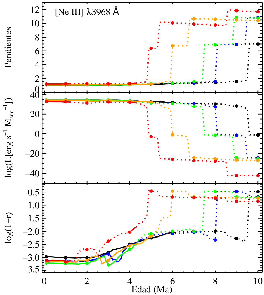
FIGURA A.5: Pendientes, \log L(1 M_{\odot}) y \log(1-r) para [Ne III] \lambda 3968 \text{ \AA} .
