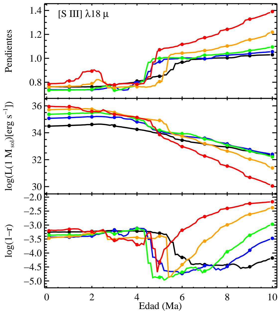
FIGURA B.32: Pendientes, \log L(1 M_{\odot}) y \log(1-r) para [S III] \lambda 18 \mu .
