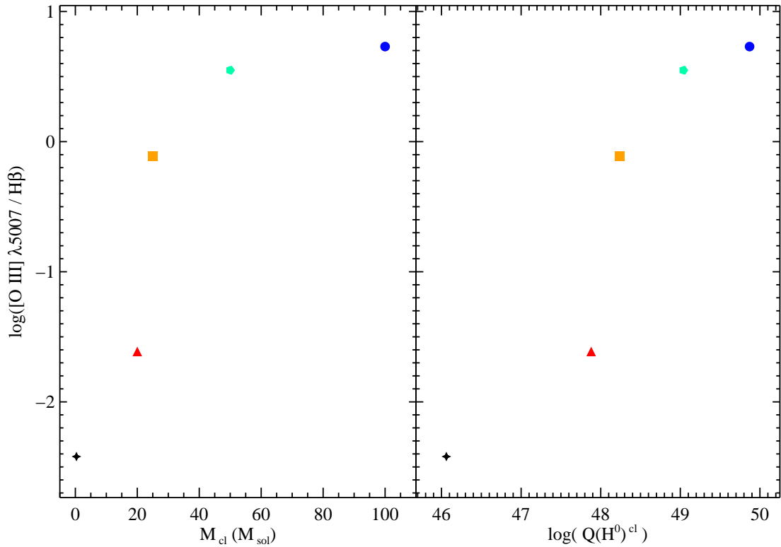
FIGURA 2.5: Intensidad de la línea [O\ III]\ \lambda\ 5007\ \text{\AA} con respecto a H\beta frente a la masa del cúmulo (izquierda) y al número de fotones ionizantes (derecha) para las simulaciones del escenario de número de estrellas fijo. Estrella negra: simulación con modelo de síntesis; Triángulo rojo: simulación con estrella de 20\ M_{\odot} ; Cuadrado naranja: simulación con estrella de 25\ M_{\odot} ; Pentágono verde: simulación con estrella de 50\ M_{\odot} ; Círculo azul: simulación con estrella de 100\ M_{\odot} .
