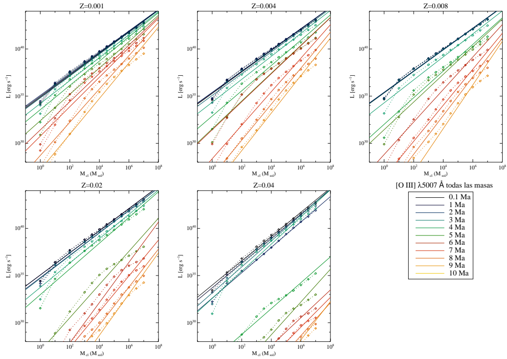
FIGURA 4.5: Regresiones completas para [O III] \lambda 5007 Å. Símbolos como en Fig. 4.3.
