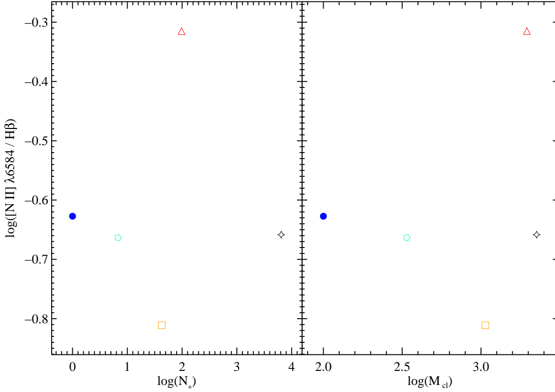
FIGURA 2.12: Igual que la Fig. 2.11 para la línea [N II] \lambda 6584 Å.
