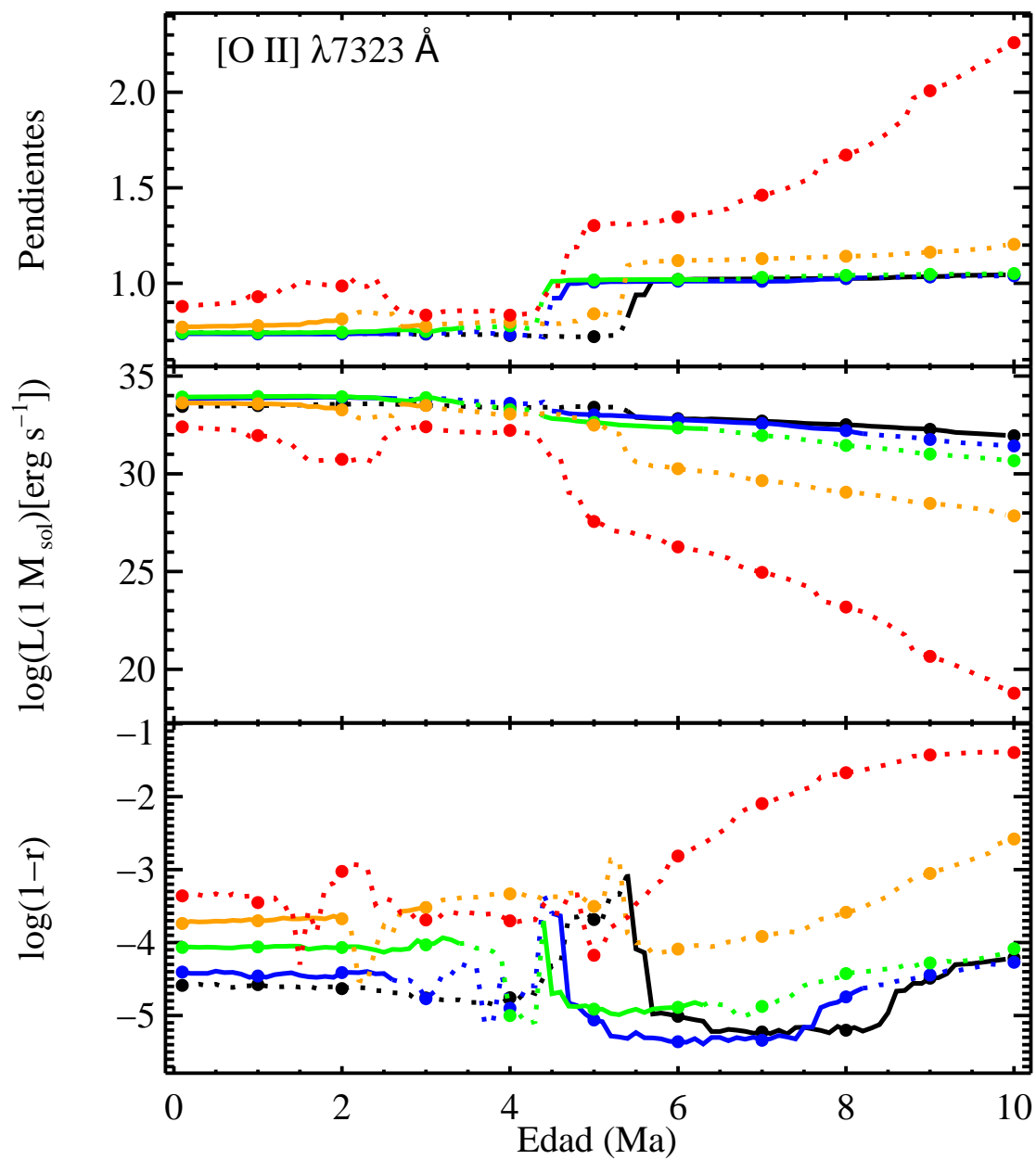
FIGURA B.23: Pendientes, \log L(1 M_{\odot}) y \log(1-r) para [O II] \lambda 7323 Å.
