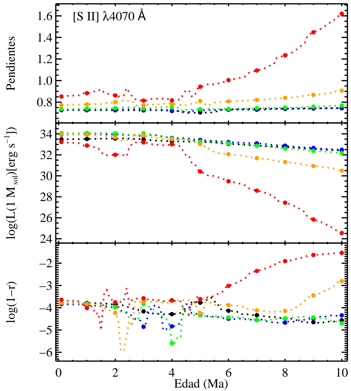
FIGURA B.6: Pendientes, \log L(1 M_{\odot}) y \log(1-r) para [S \text{ II}] \lambda 4070 \text{ \AA} .
