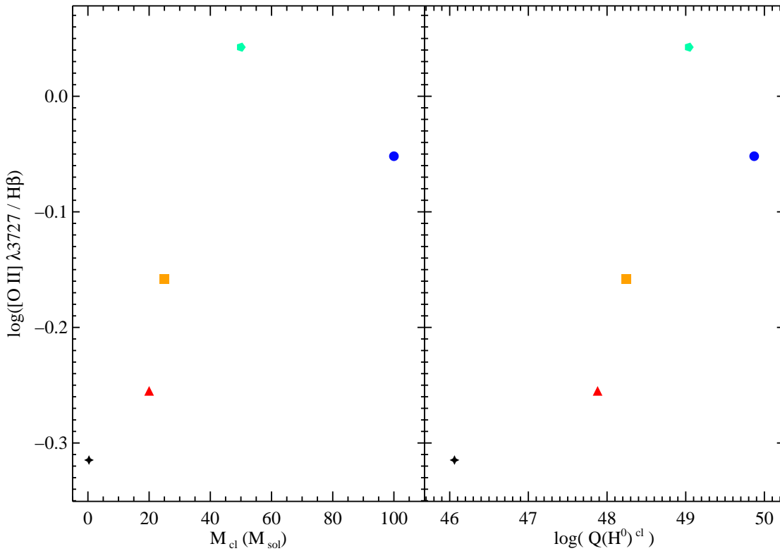
FIGURA 2.6: Igual que la Fig. 2.5 para la línea [O II] \lambda 3727 Å.
