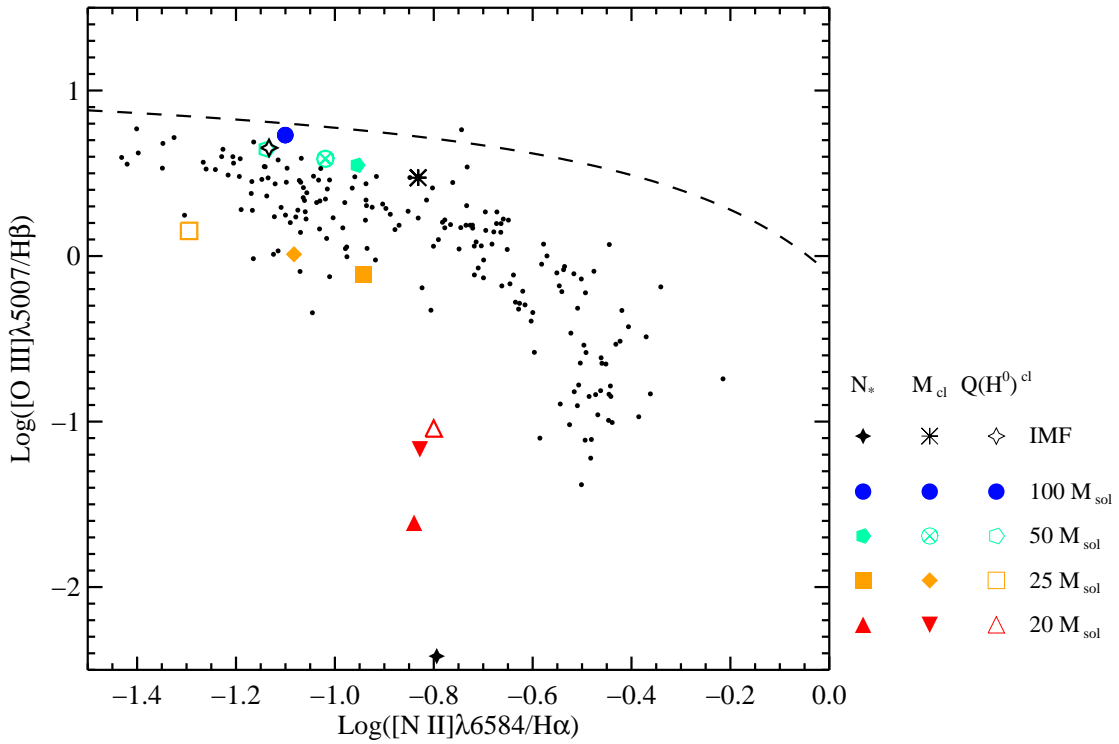
FIGURA 2.13: Diagrama de diagnóstico [O III] 5007/H\beta vs. [N II] 6584/H\alpha donde se comparan las simulaciones realizadas con los datos de van Zee et al. (1998) (puntos negros). Con trazo discontinuo se muestra el límite teórico de la zona cubierta por regiones H II propuesta por Kewley et al. (2001).
