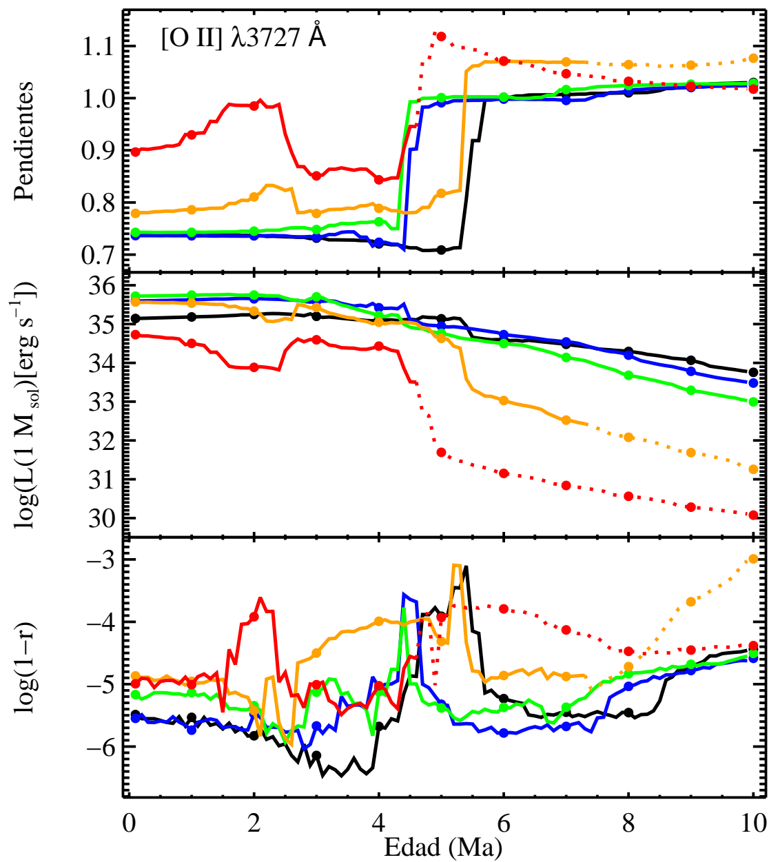
FIGURA B.2: Pendientes, \log L(1 M_{\odot}) y \log(1-r) para [O II] \lambda 3727 \text{ \AA} .
