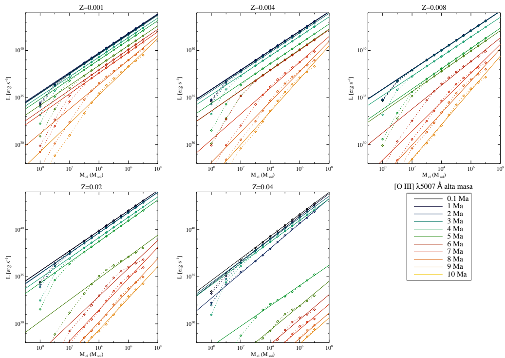
FIGURA 4.6: Regresiones de alta masa para [O III] \lambda 5007 Å. Símbolos como en Fig. 4.3.
