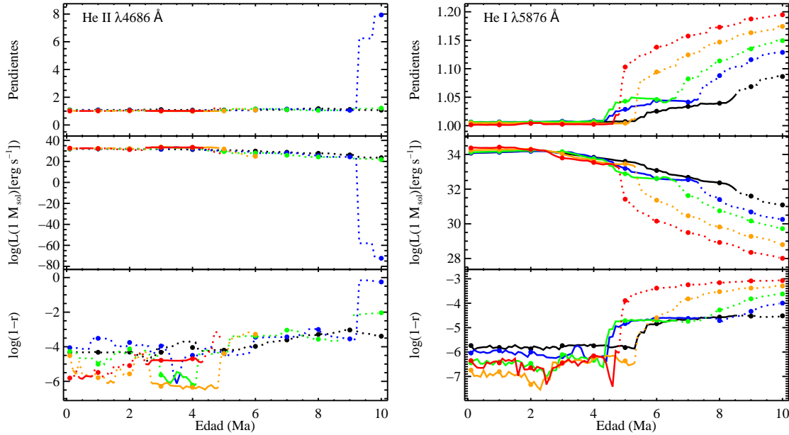
FIGURA 4.4: Resultados de las regresiones de alta masa para He II \lambda 4686 \text{ \AA} y He I \lambda 5876 \text{ \AA} . En línea discontinua se muestran las edades para las cuales no se cumple el criterio de visibilidad de EW_{\text{SR}} \geq 1 \text{ \AA} . Colores como en Fig. 4.1.
