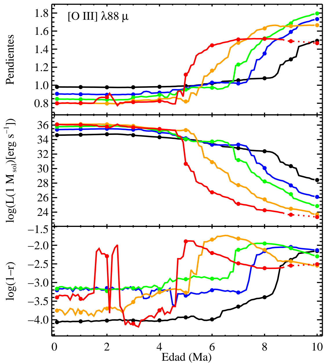
FIGURA B.37: Pendientes, \log L(1 M_{\odot}) y \log(1-r) para [O III] \lambda 88 \mu .
