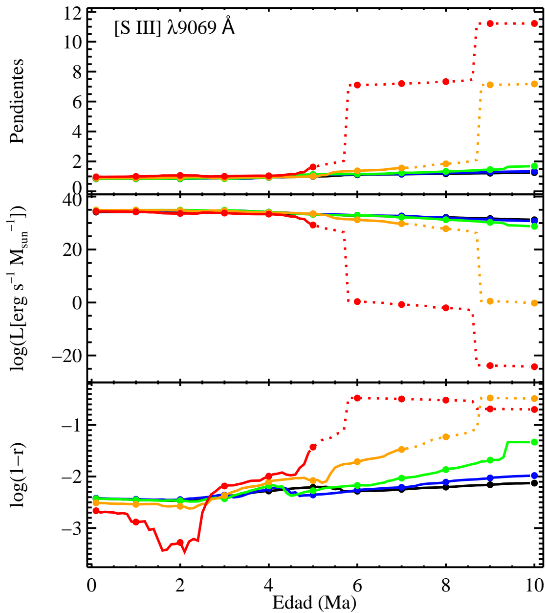
FIGURA A.25: Pendientes, \log L(1 M_{\odot}) y \log(1-r) para [S \text{ III}] \lambda 9069 \text{ \AA} .
