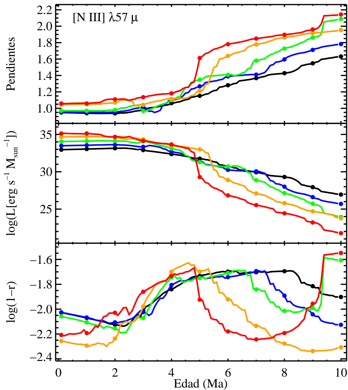
FIGURA A.36: Pendientes, \log L(1 M_{\odot}) y \log(1-r) para [\text{N III}] \lambda 57 \mu .
