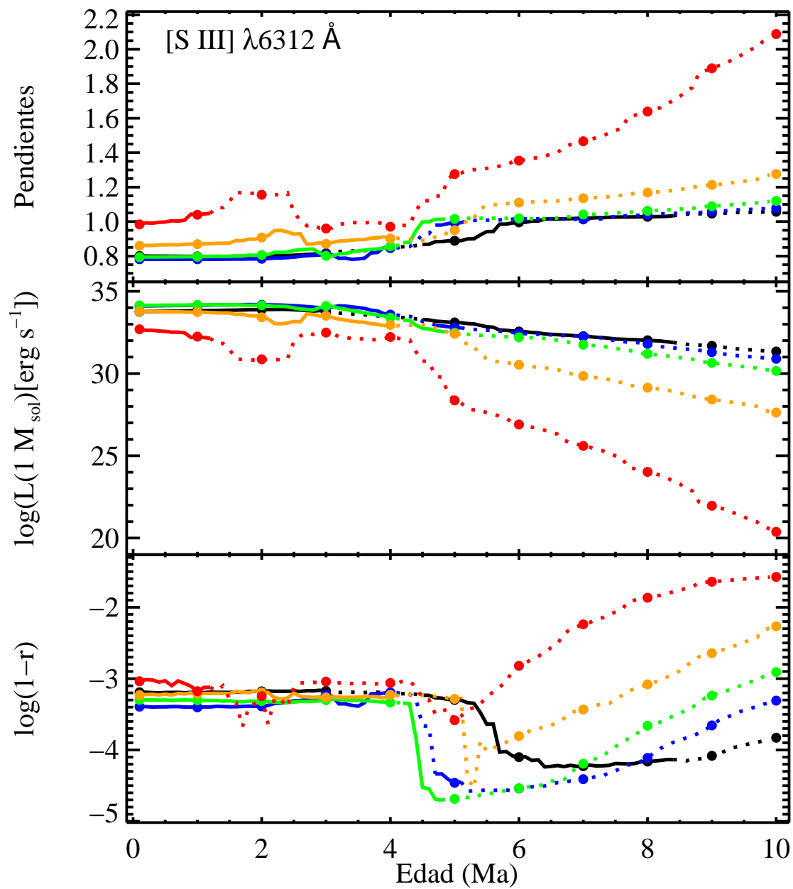
FIGURA B.15: Pendientes, \log L(1 M_{\odot}) y \log(1-r) para [S III] \lambda 6312 Å.
