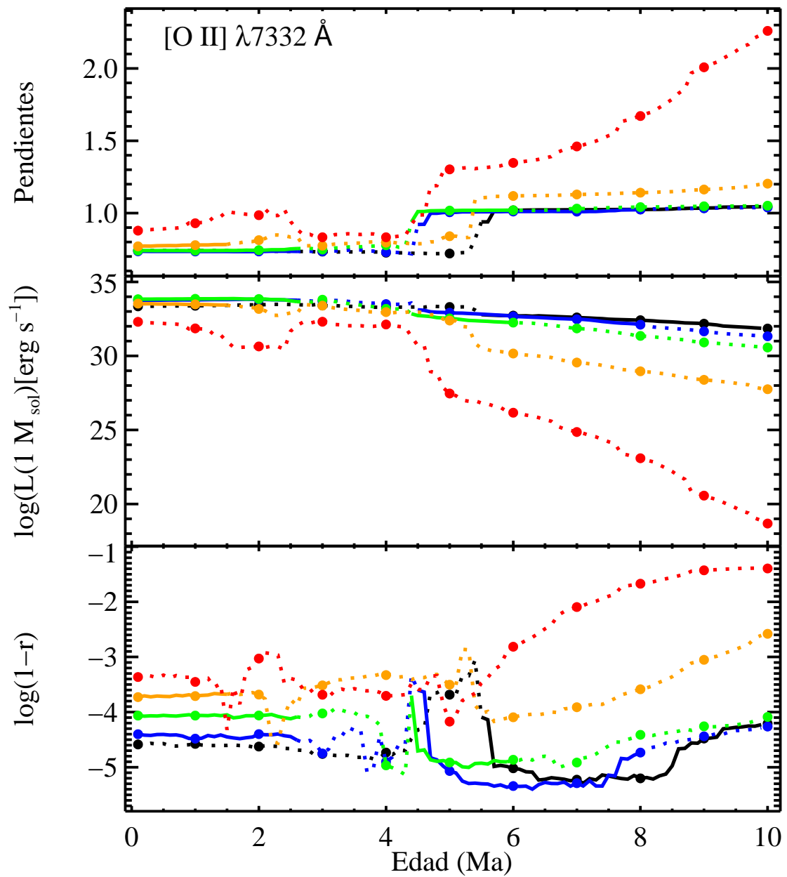
FIGURA B.24: Pendientes, \log L(1 M_{\odot}) y \log(1-r) para [O II] \lambda 7332 \text{ \AA} .
