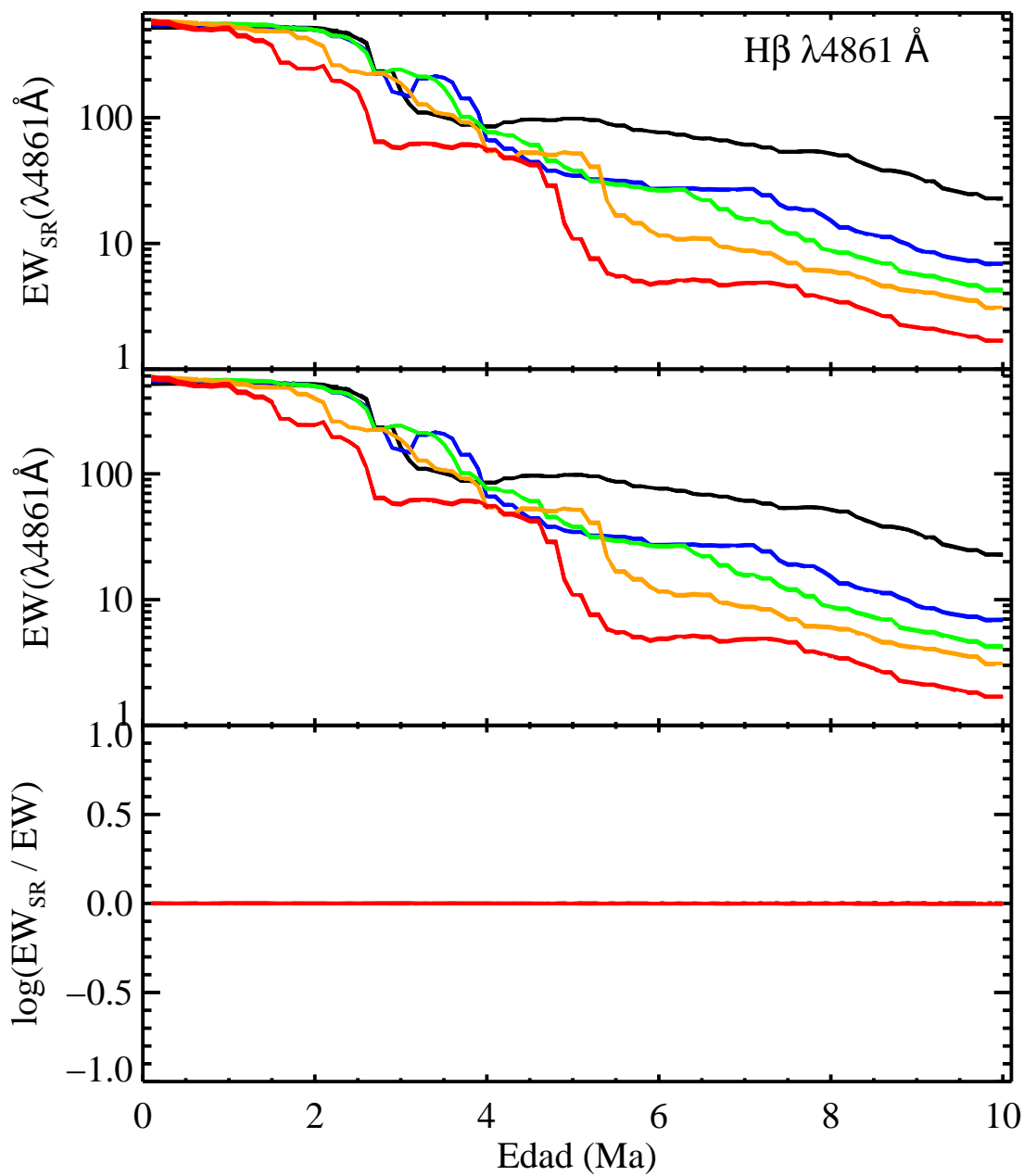
FIGURA C.10: EW_{SR} , EW y \log \frac{EW_{SR}}{EW} para H \beta .
