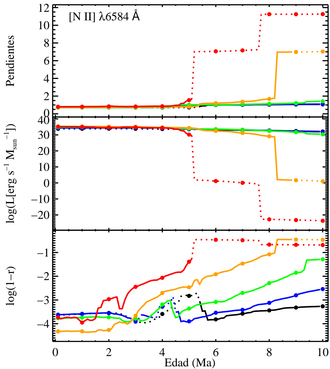
FIGURA A.18: Pendientes, \log L(1 M_{\odot}) y \log(1-r) para [\text{N II}] \lambda 6584 \text{ \AA} .
