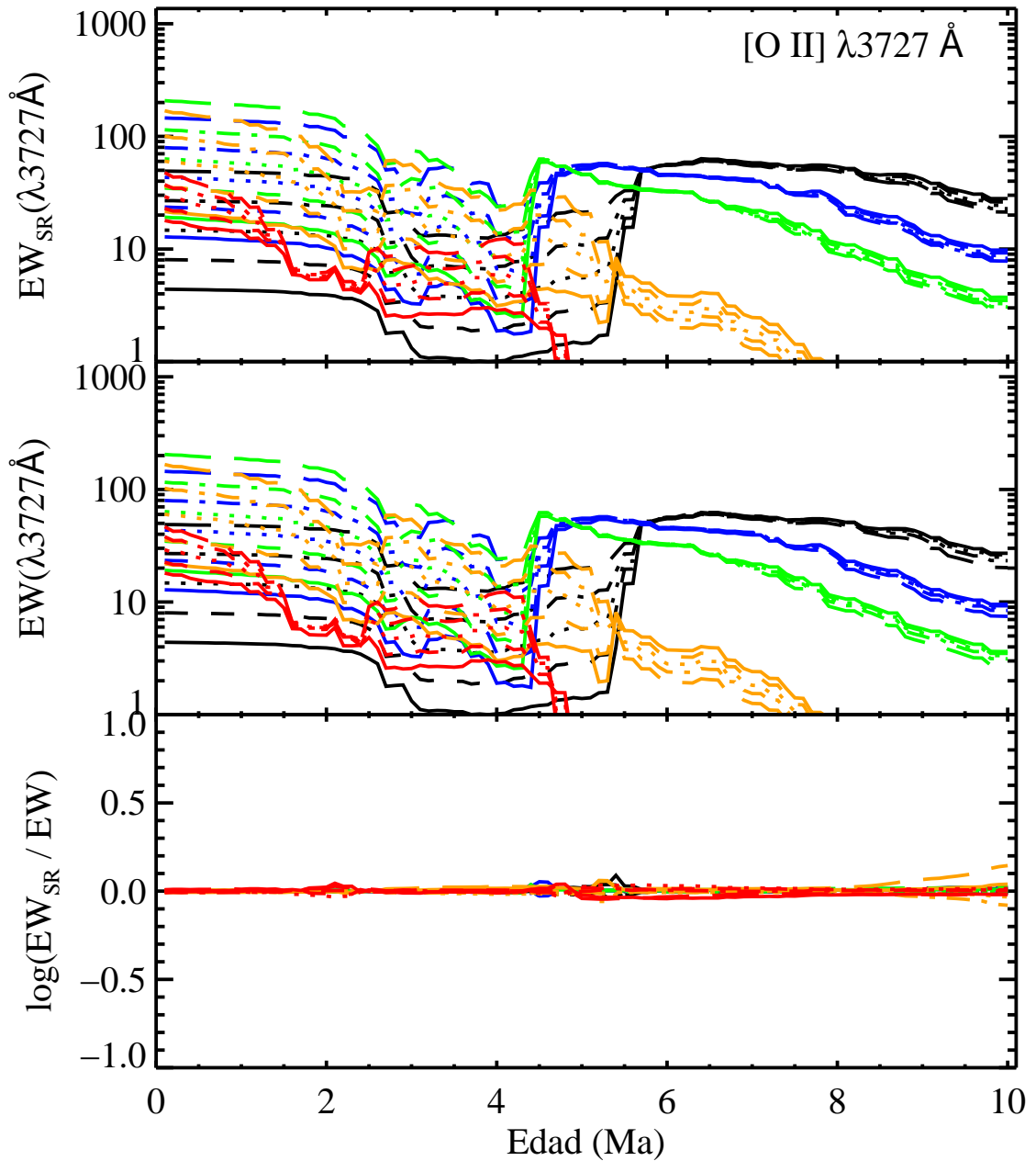
FIGURA 4.14: Anchuras equivalentes de la línea [O II] \lambda 3727 \text{ \AA} . Disposición y símbolos como en Fig. 4.12.
