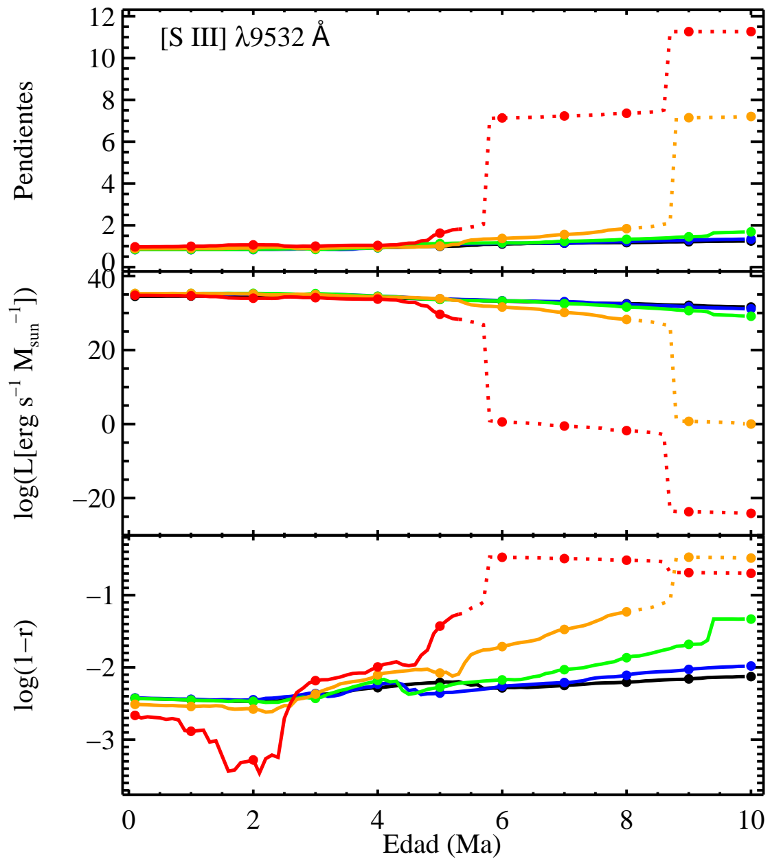
FIGURA A.26: Pendientes, \log L(1 M_{\odot}) y \log(1-r) para [S III] \lambda 9532 Å.
