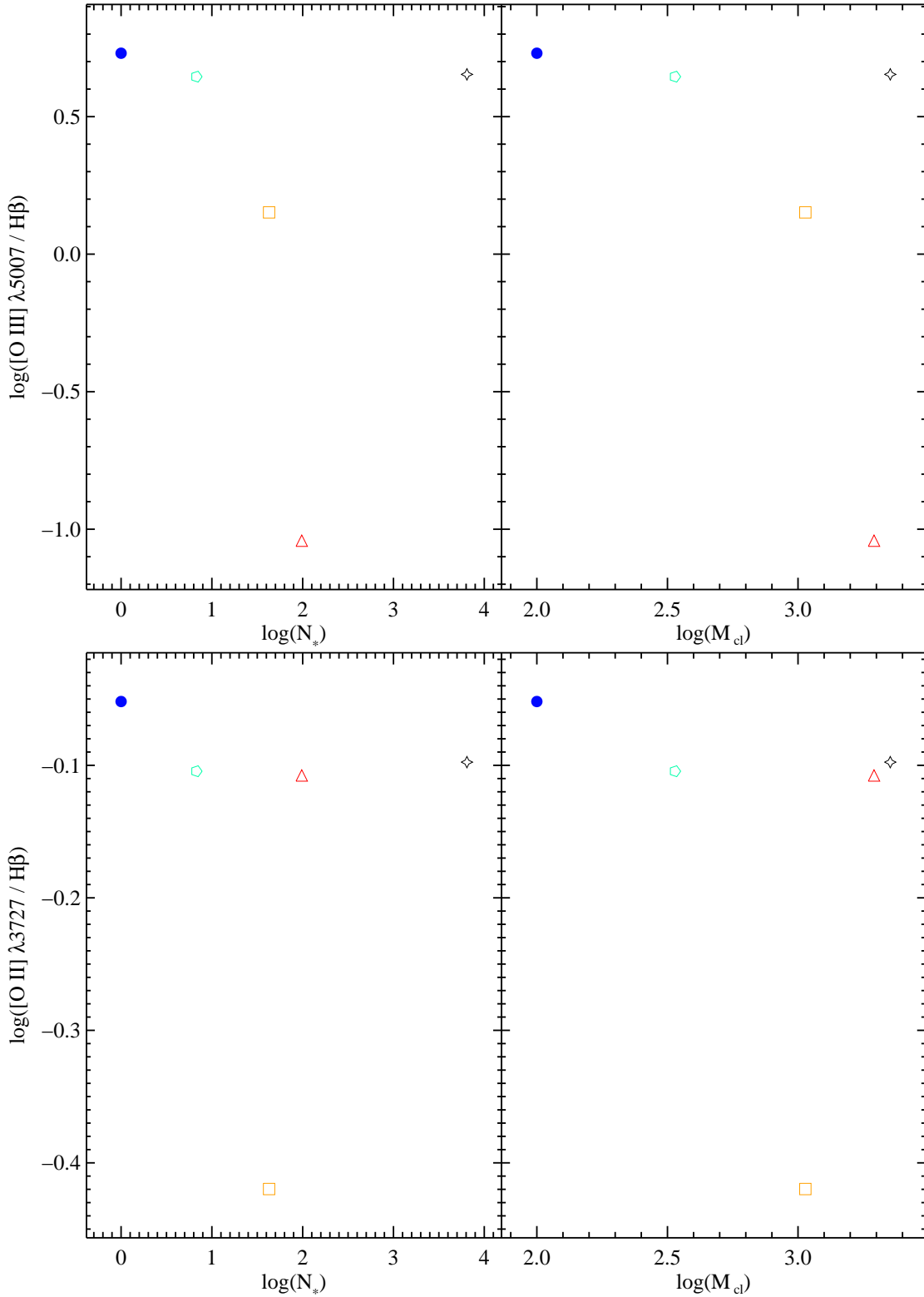
FIGURA 2.11: Intensidades de [O\ III] \lambda 5007 \text{ \AA} (arriba) y [O\ II] \lambda 3727 \text{ \AA} (abajo) con respecto a H\beta frente al número total de estrellas en el cúmulo (izquierda) y a la masa del cúmulo (derecha) para las simulaciones del escenario de número de fotones ionizantes fijo. Estrella negra hueca: simulación con modelo de síntesis; Triángulo rojo hueco: simulación con estrellas de 20 M_{\odot} ; Cuadrado naranja hueco: simulación con estrellas de 25 M_{\odot} ; Pentágono verde hueco: simulación con estrellas de 50 M_{\odot} ; Círculo azul: simulación con estrella de 100 M_{\odot} .
