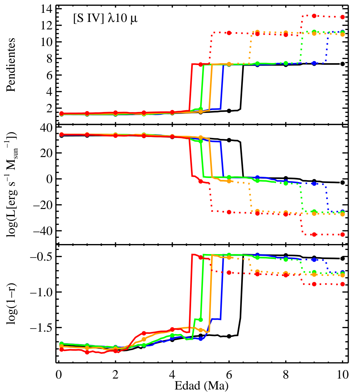
FIGURA A.29: Pendientes, \log L(1 M_{\odot}) y \log(1-r) para [S \text{ IV}] \lambda 10 \mu .
