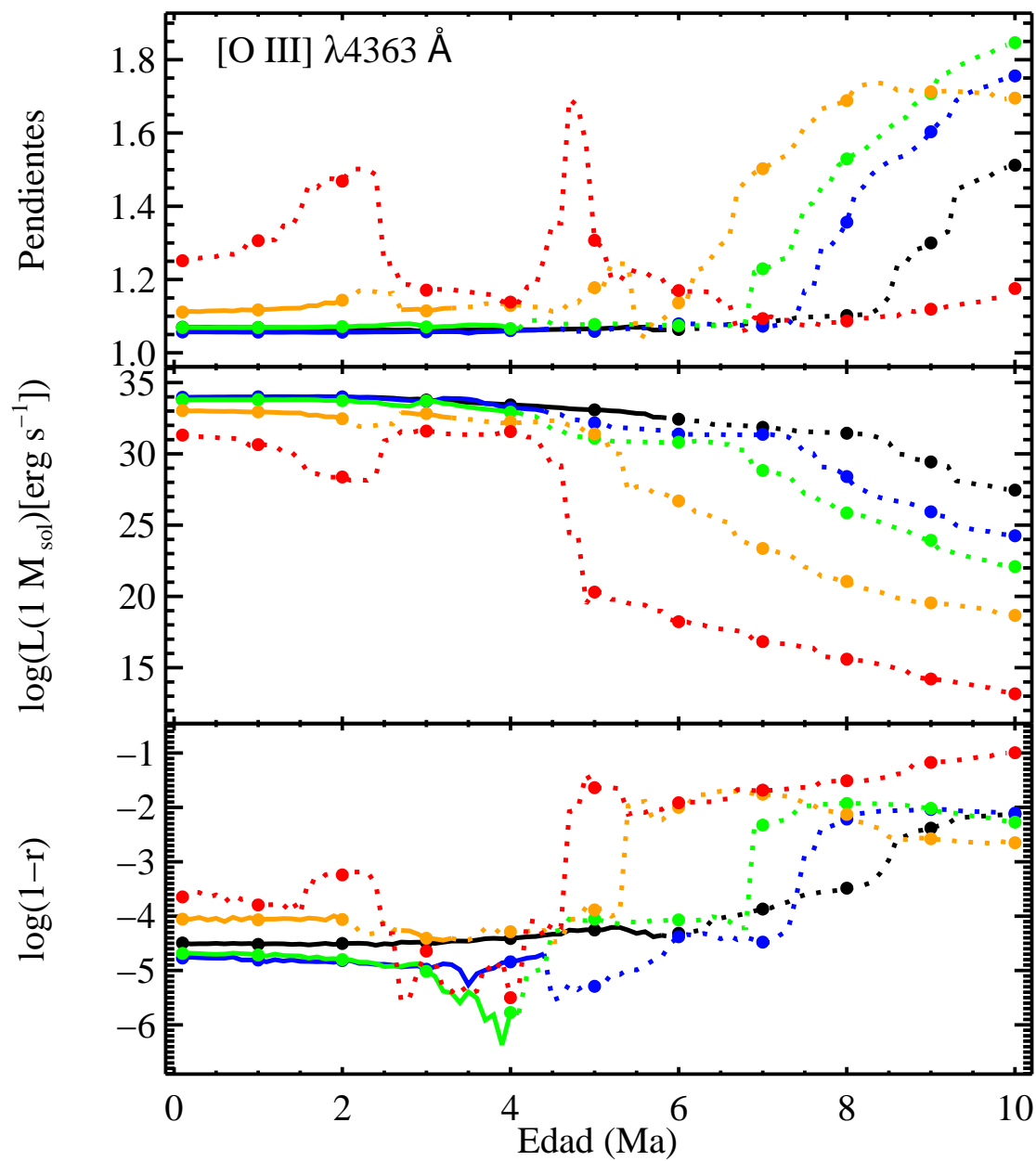
FIGURA B.8: Pendientes, \log L(1 M_{\odot}) y \log(1-r) para [O III] \lambda 4363 Å.
