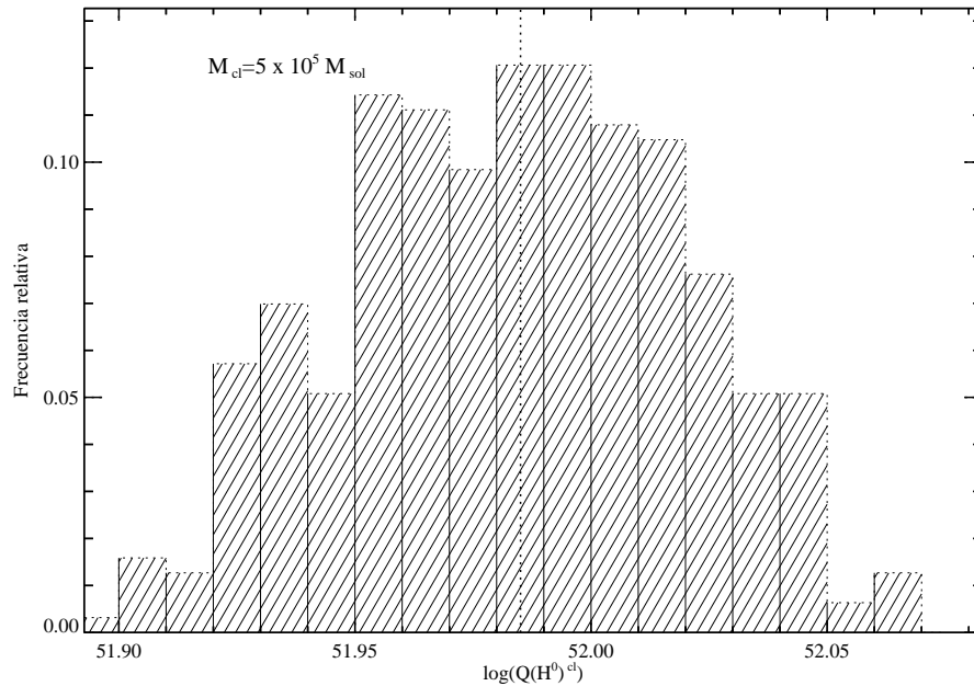
FIGURA 3.9: Distribución de \log Q(H^0)^{cl} para simulaciones con M_{cl} \approx 5 \times 10^5 M_{\odot} . La línea vertical muestra el valor medio \log(Q(H^0)^{cl}) = 51.98 de la distribución.
