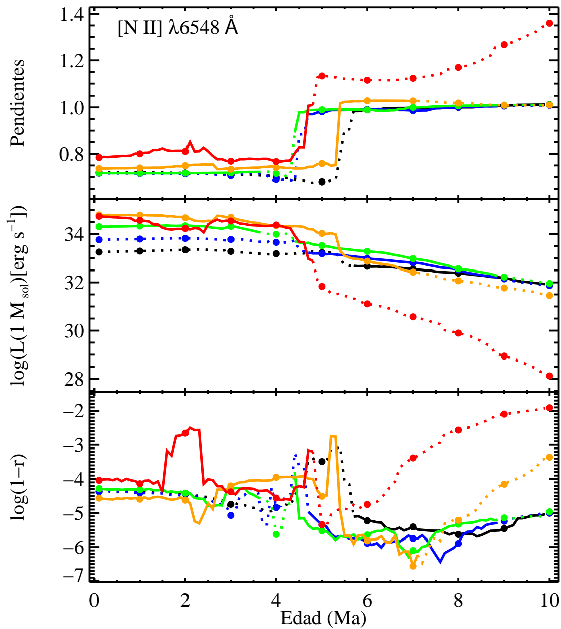
FIGURA B.16: Pendientes, \log L(1 M_{\odot}) y \log(1-r) para [N II] \lambda 6548 \text{ \AA} .
