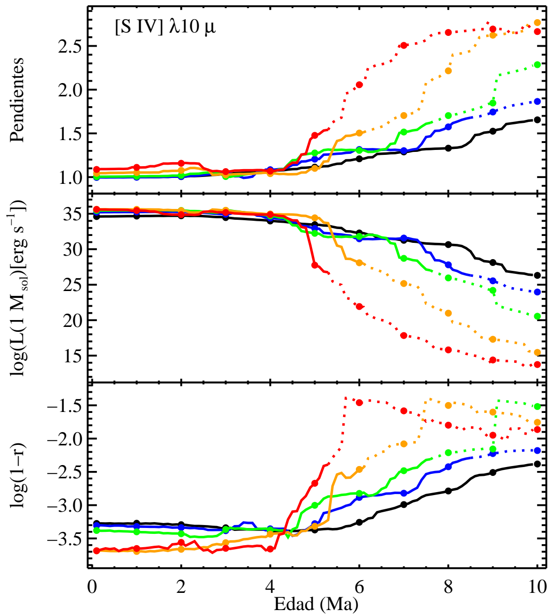
FIGURA B.29: Pendientes, \log L(1 M_{\odot}) y \log(1-r) para [S IV] \lambda 10 \mu .
