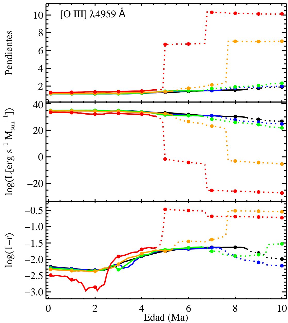
FIGURA A.11: Pendientes, \log L(1 M_{\odot}) y \log(1-\tau) para [O III] \lambda 4959 Å.
