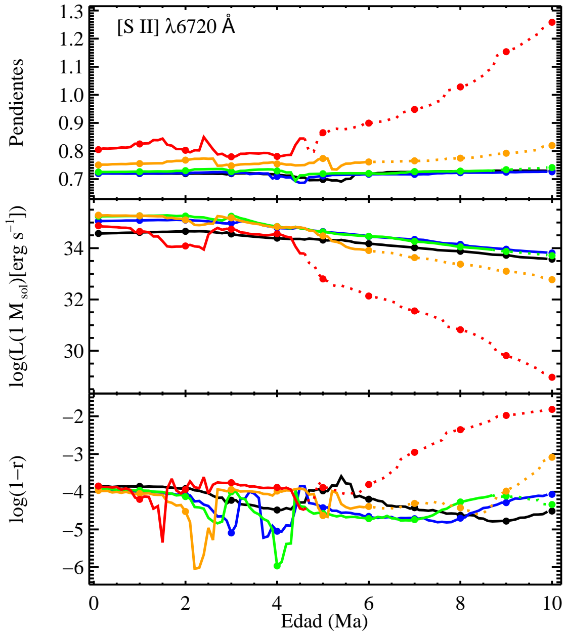
FIGURA B.20: Pendientes, \log L(1 M_{\odot}) y \log(1-r) para [S II] \lambda 6720 \text{ \AA} .
