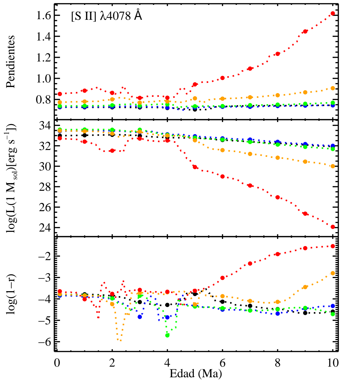
FIGURA B.7: Pendientes, \log L(1 M_{\odot}) y \log(1-r) para [S II] \lambda 4078 \text{ \AA} .
