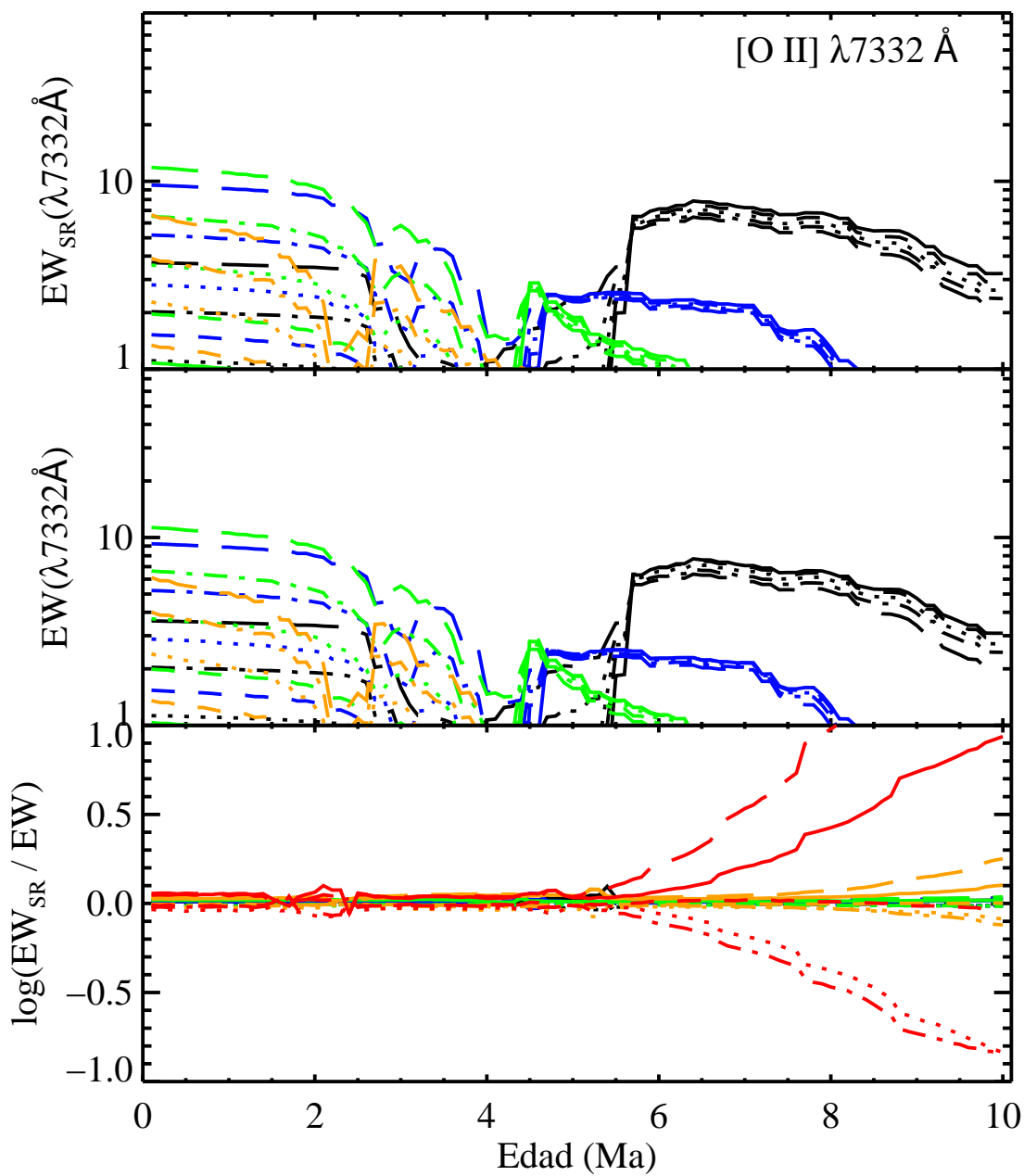
FIGURA C.24: EW_{SR} , EW y \log \frac{EW_{SR}}{EW} para [O II] \lambda 7332 Å.
