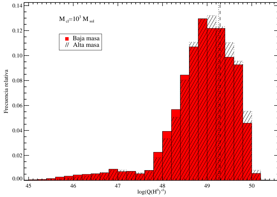
FIGURA 3.8: Distribución de \log Q(H^0)^{cl} para simulaciones con M_{cl} \approx 10^3 M_{\odot} . La línea vertical discontinua muestra el valor medio \log(Q(H^0)^{cl}) = 49.29 de la distribución obtenido con las simulaciones del conjunto de alta masa, mientras que la punteada muestra el valor medio \log(Q(H^0)^{cl}) = 49.26 obtenido con el conjunto de baja masa y con color sólido se muestran los valores correspondientes al conjunto de baja masa y con trama rayada los correspondientes al de alta masa.
