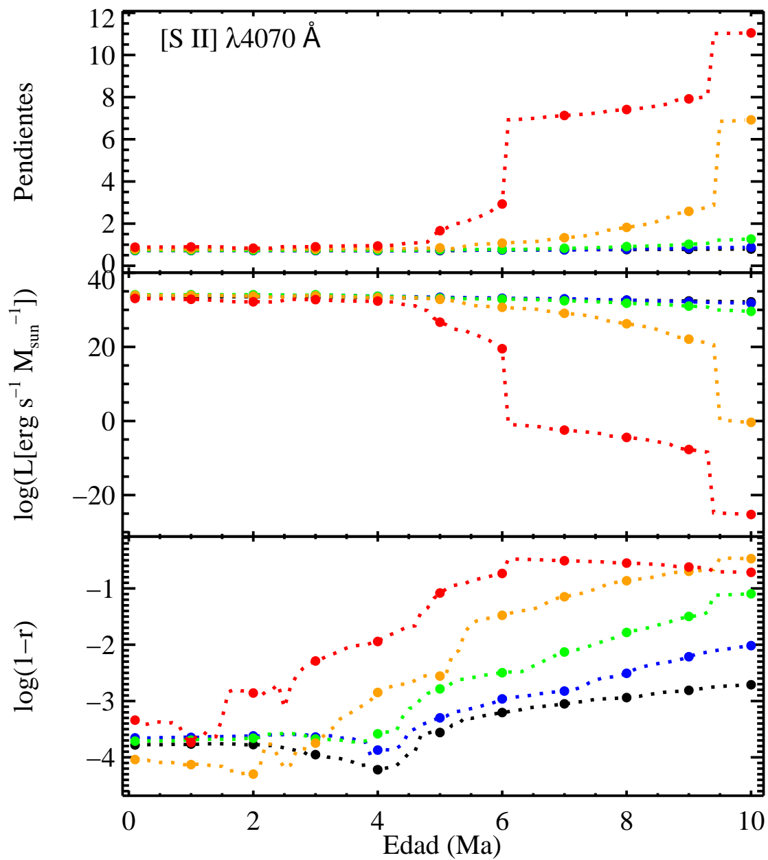
FIGURA A.6: Pendientes, \log L(1 M_{\odot}) y \log(1-r) para [S II] \lambda 4070 Å.
