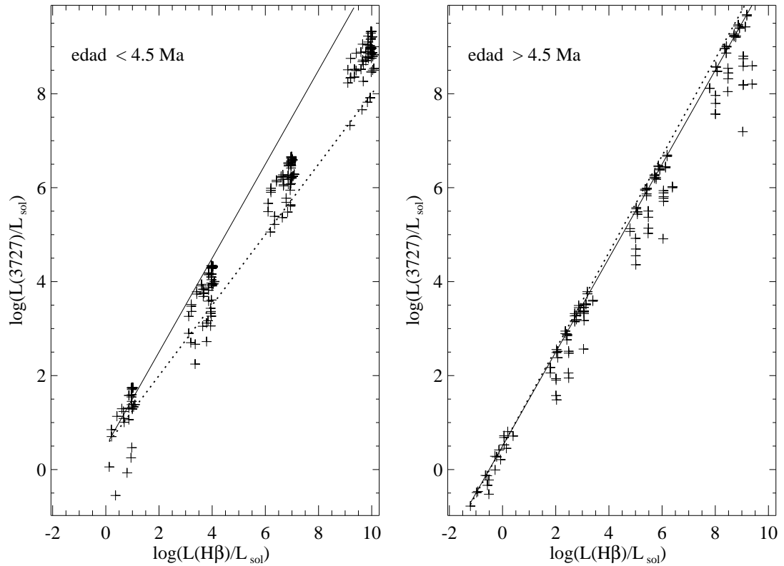
FIGURA 4.26: Luminosidad de [O II] \lambda 3727 \text{ \AA} frente a la luminosidad de H\beta para los modelos de Stasińska et al. (2001) con edades menores (izquierda) y mayores (derecha) que 4.5 Ma. Como referencia se muestran una línea con pendiente igual a 1 (línea continua) y líneas con las pendientes características de la línea de emisión en cada rango de edad (línea discontinua).
