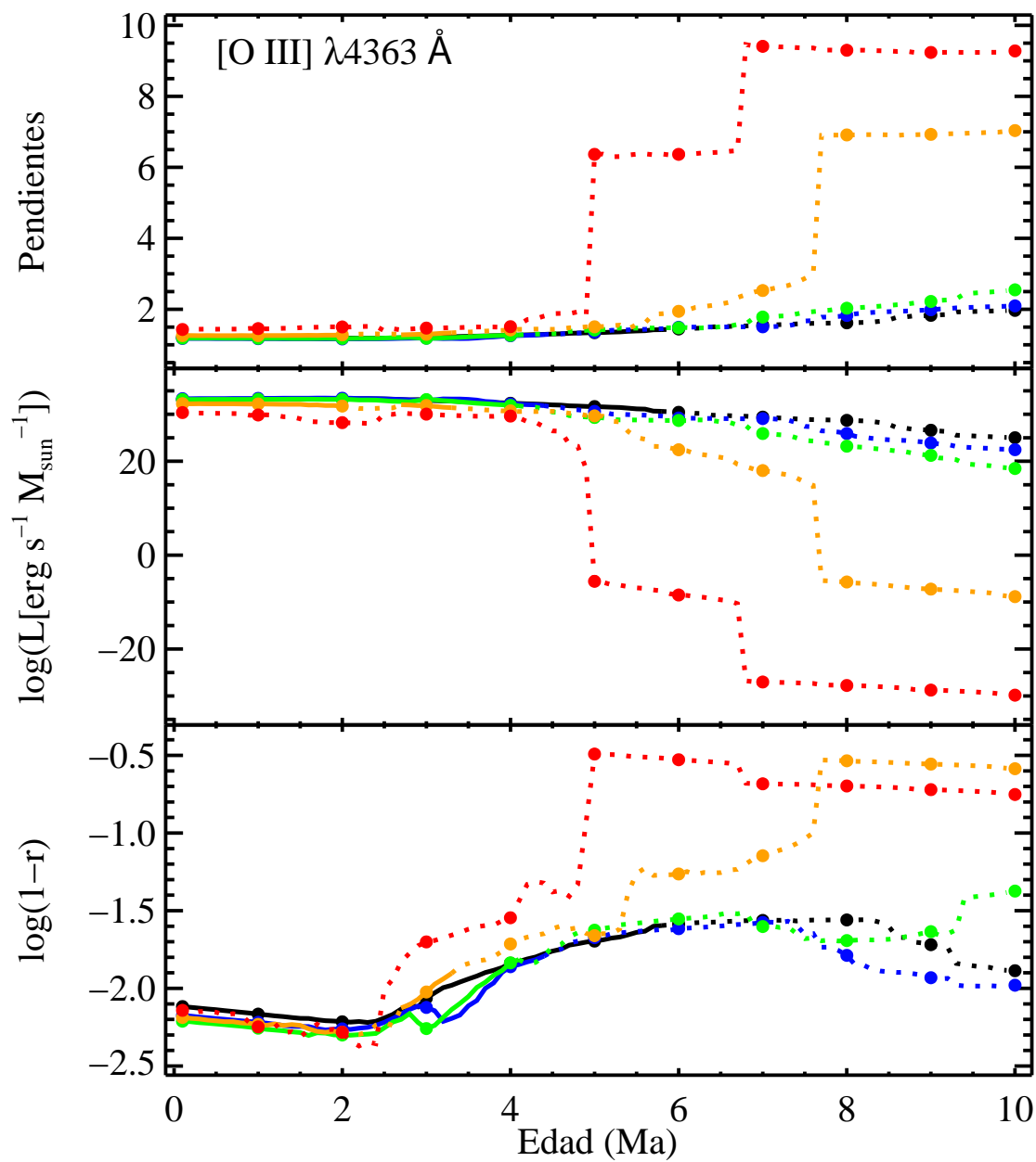
FIGURA A.8: Pendientes, \log L(1 M_{\odot}) y \log(1-r) para [O III] \lambda 4363 Å.
