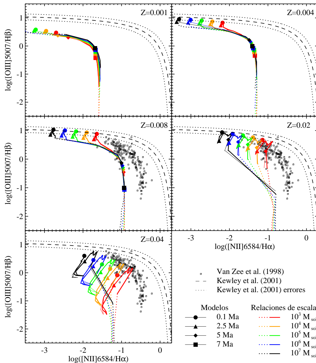
FIGURA 4.18: Diagrama de diagnóstico de [\text{O III}] 5007/\text{H}\beta frente a [\text{N II}] 6584/\text{H}\alpha para cada metalicidad. Los colores representan la masa de cúmulo. Líneas finas: resultados de los modelos, líneas gruesas: resultados de relaciones de escala, línea gruesa discontinua: resultados de relaciones de escala que no cumplen el criterio de visibilidad ( EW_{\text{SR}} \geq 1 \text{ \AA} ). Con símbolos sólidos superpuestos a las curvas de los modelos se representan los resultados para cuatro edades de referencia (círculo: 0.1 Ma; triángulo: 2.5 Ma; rombo: 5 Ma; cuadrado: 7 Ma). Como referencia se muestran también las observaciones de van Zee et al. (1998) (cuadrados negros huecos), y la curva de Kewley et al. (2001) (línea rayada negra) con sus límites de error (línea punteada negra).
