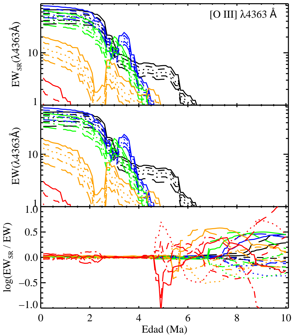
FIGURA C.8: EW_{SR} , EW y \log \frac{EW_{SR}}{EW} para [O III] \lambda 4363 Å.
