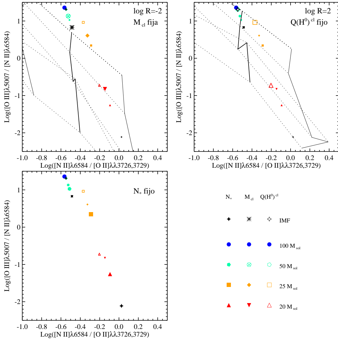
FIGURA 2.16: Diagramas de diagnóstico [\text{O III}] 5007/[\text{N II}] 6584 frente a [\text{N II}] 6584/[\text{O II}] 3726, 3729 . Símbolos como en Fig. 2.14.
