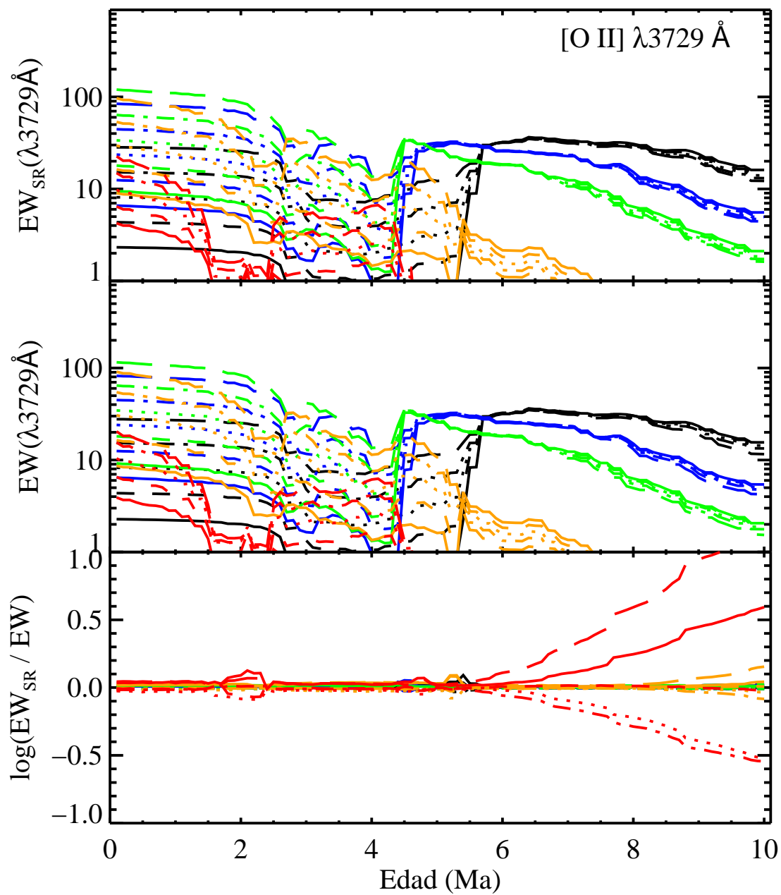
FIGURA C.3: EW_{SR} , EW y \log \frac{EW_{SR}}{EW} para [O II] \lambda 3729 \text{ \AA} .
