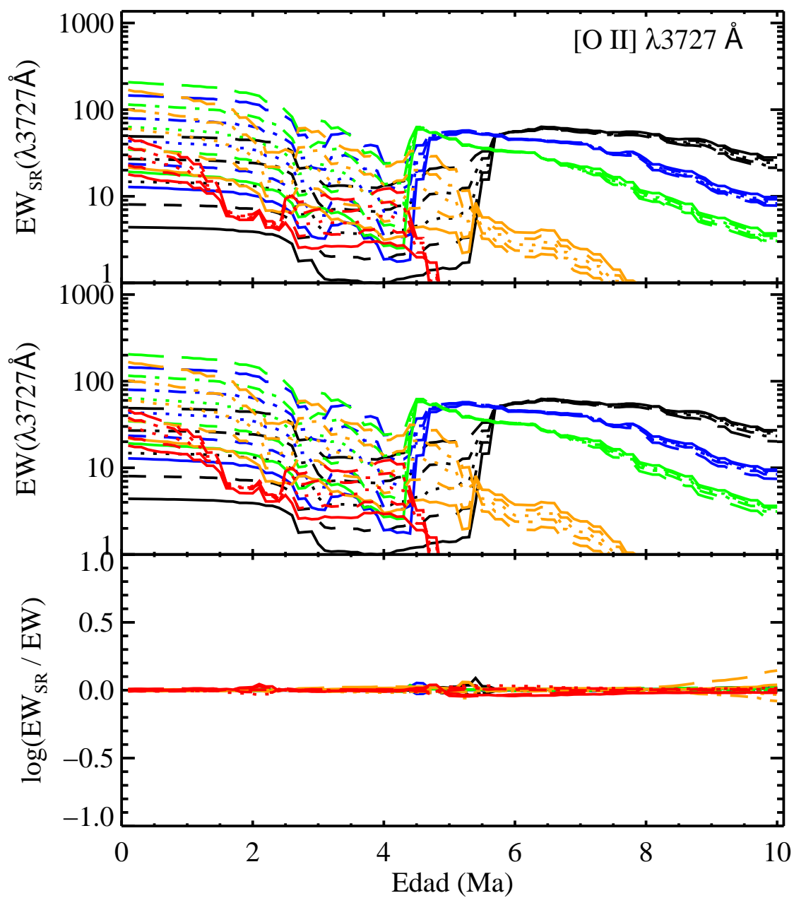
FIGURA C.2: EW_{SR} , EW y \log \frac{EW_{SR}}{EW} para [O II] \lambda 3727 \text{ \AA} .
