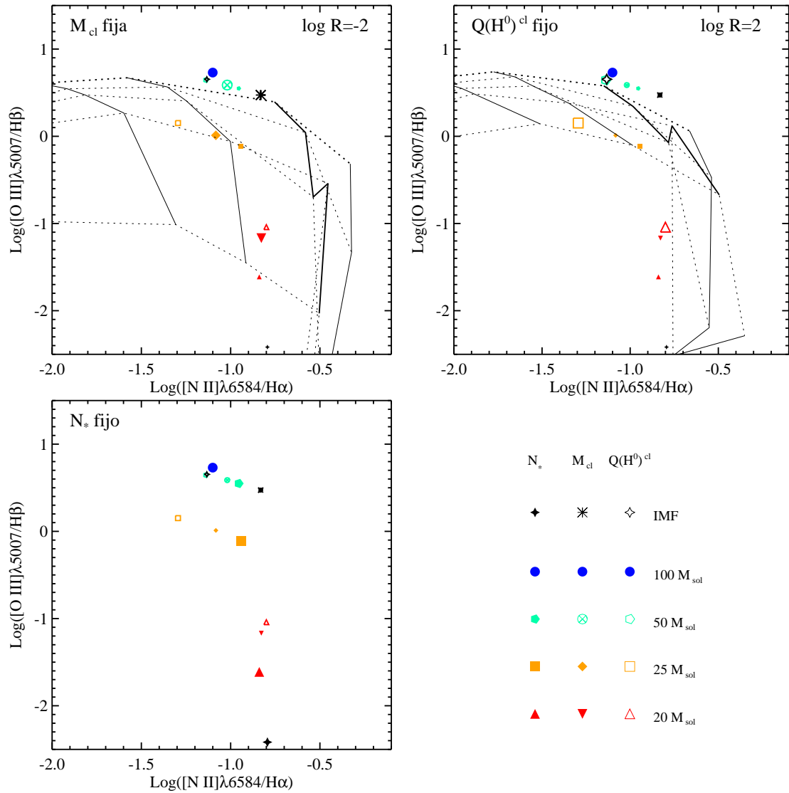
FIGURA 2.14: Diagramas de diagnostico [\text{O III}] 5007/\text{H}\beta vs. [\text{N II}] 6584/\text{H}\alpha , donde resaltamos en cada gráfica uno de los tres escenarios considerados aumentando el tamaño de los símbolos correspondientes. En las gráficas correspondientes a los escenarios de M_{cl} fija y Q(H^0)^{cl} fija se incluyen la malla de Dopita et al. (2006a) que mejor ajusta (ver texto). Líneas continuas: curvas de igual metalicidad. Líneas discontinuas: curvas de igual edad. En trazo grueso se destacan las curvas correspondientes a Z_{\odot} y edad 0.2 Ma.
