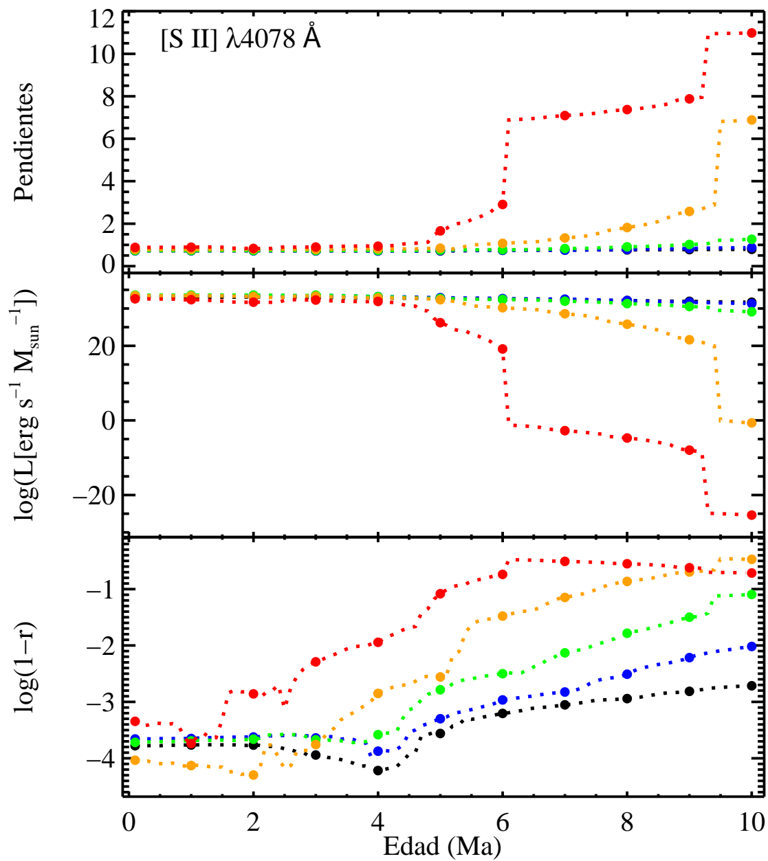
FIGURA A.7: Pendientes, \log L(1 M_{\odot}) y \log(1-r) para [S II] \lambda 4078 \text{ \AA} .
