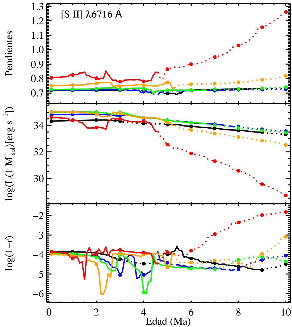
FIGURA B.19: Pendientes, \log L(1 M_{\odot}) y \log(1-r) para [S II] \lambda 6716 \text{ \AA} .
