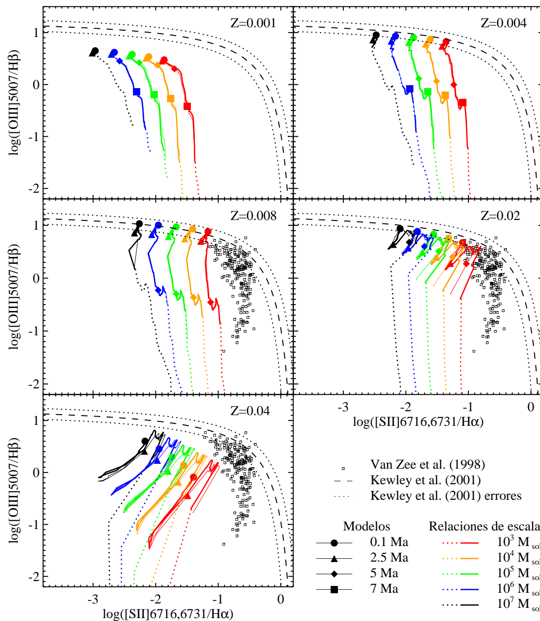
FIGURA 4.19: Diagrama de diagnóstico de [\text{O III}] 5007/\text{H}\beta frente a [\text{S II}] 6716,6731/\text{H}\alpha para cada metalicidad. Los símbolos tienen el mismo significado que en la Fig. 4.18.
