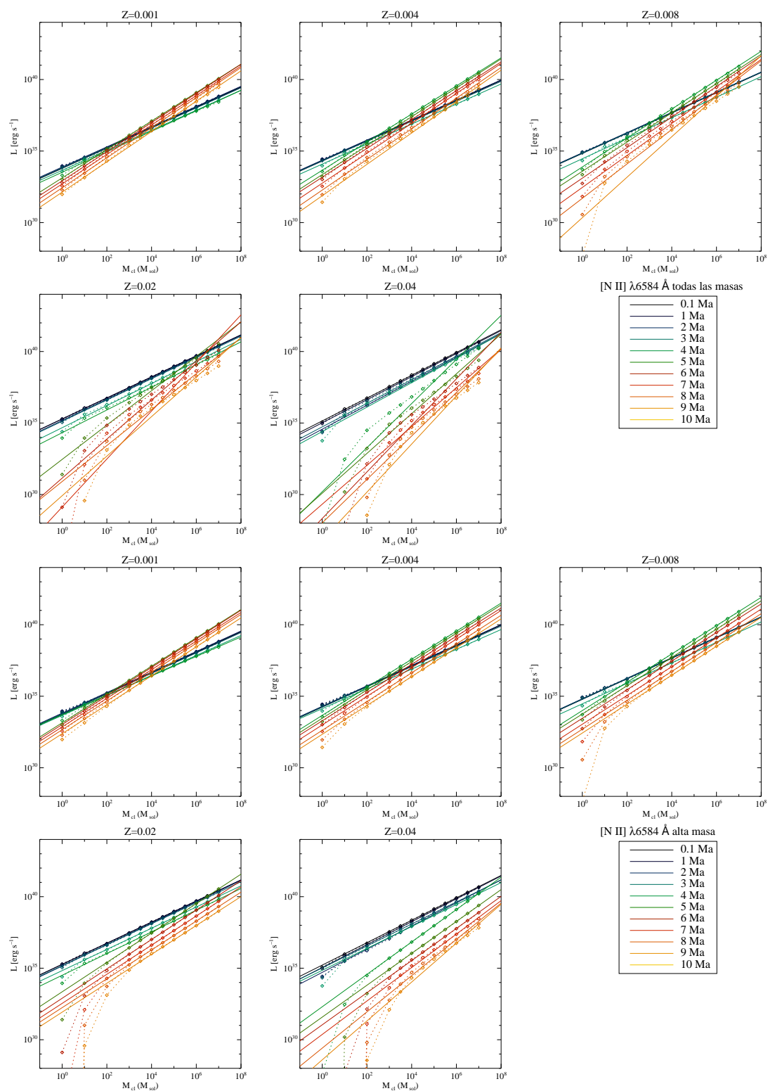
FIGURA 4.9: Regresiones completas y de alta masa para [N II] \lambda 6584 \text{ \AA} . Símbolos como en Fig. 4.3.
