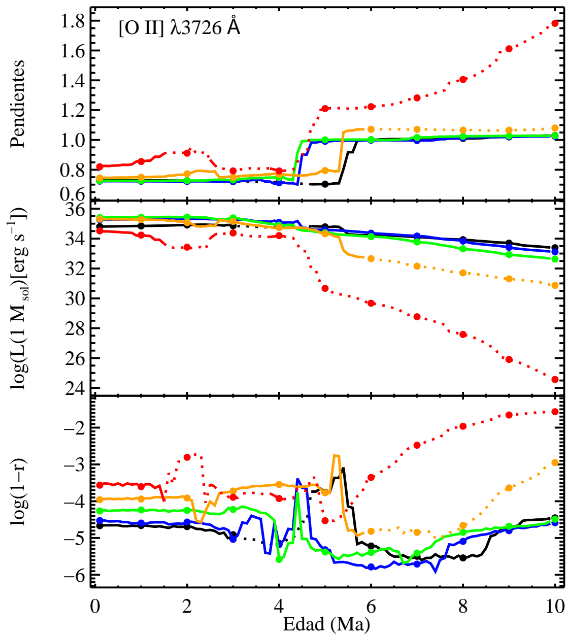
FIGURA B.1: Pendientes, \log L(1 M_{\odot}) y \log(1-r) para [O II] \lambda 3726 \text{ \AA} .
