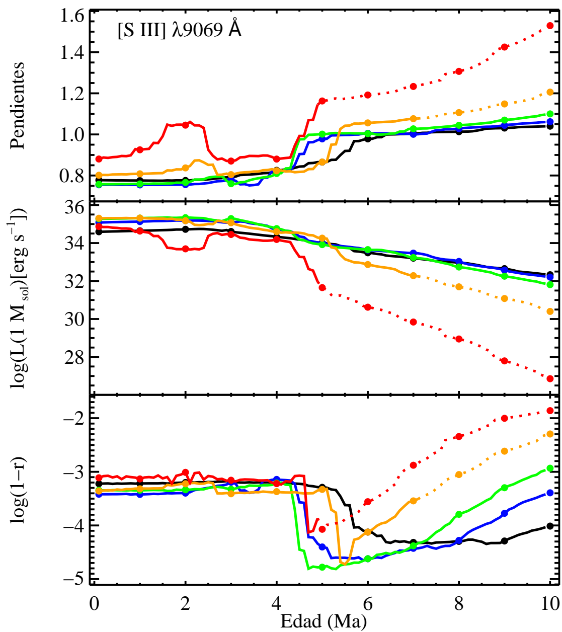
FIGURA B.25: Pendientes, \log L(1 M_{\odot}) y \log(1-r) para [S III] \lambda 9069 \text{ \AA} .
