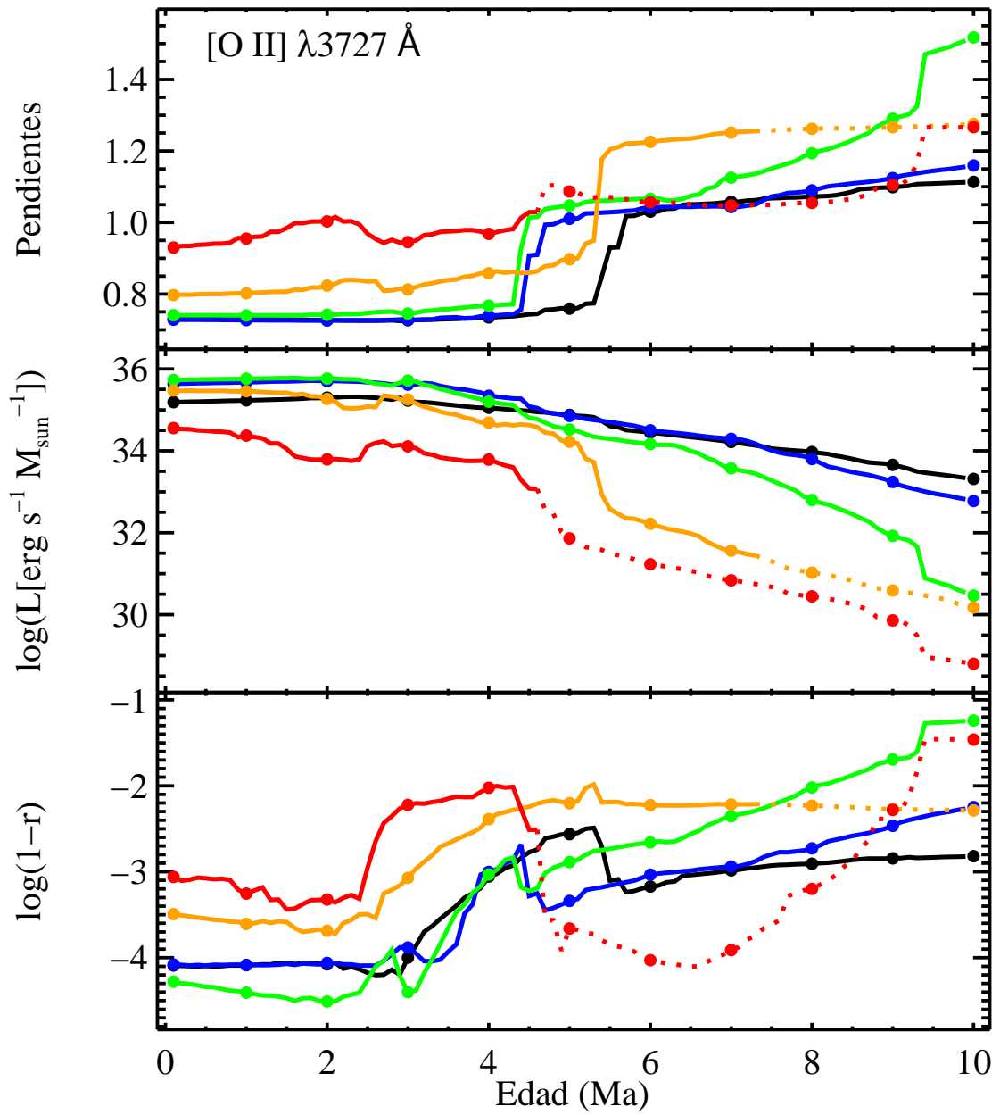
FIGURA A.2: Pendientes, \log L(1 M_{\odot}) y \log(1-r) para [\text{O II}] \lambda 3727 \text{ \AA} .
