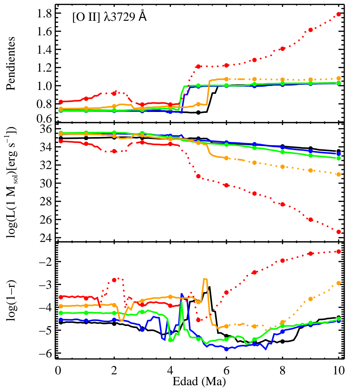
FIGURA B.3: Pendientes, \log L(1 M_{\odot}) y \log(1-r) para [O II] \lambda 3729 \text{ \AA} .
