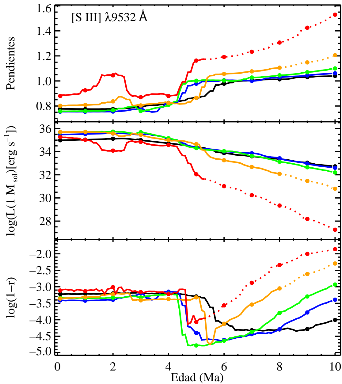
FIGURA B.26: Pendientes, \log L(1 M_{\odot}) y \log(1-r) para [S III] \lambda 9532 Å.
