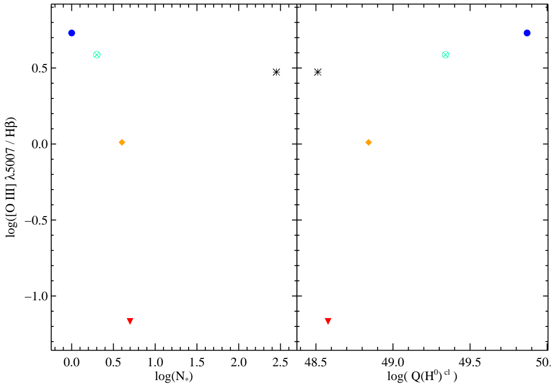
FIGURA 2.8: Intensidad de la línea [O III] \lambda 5007 Å con respecto a H \beta frente al número total de estrellas en el cúmulo (izquierda) y al número de fotones ionizantes (derecha) para las simulaciones del escenario de masa total de cúmulo fija. Asterisco: simulación con modelo de síntesis; Triángulo rojo invertido: simulación con estrellas de 20 M_{\odot} ; Diamante naranja: simulación con estrellas de 25 M_{\odot} ; Círculo con aspa verde: simulación con estrellas de 50 M_{\odot} ; Círculo azul: simulación con estrella de 100 M_{\odot} .
