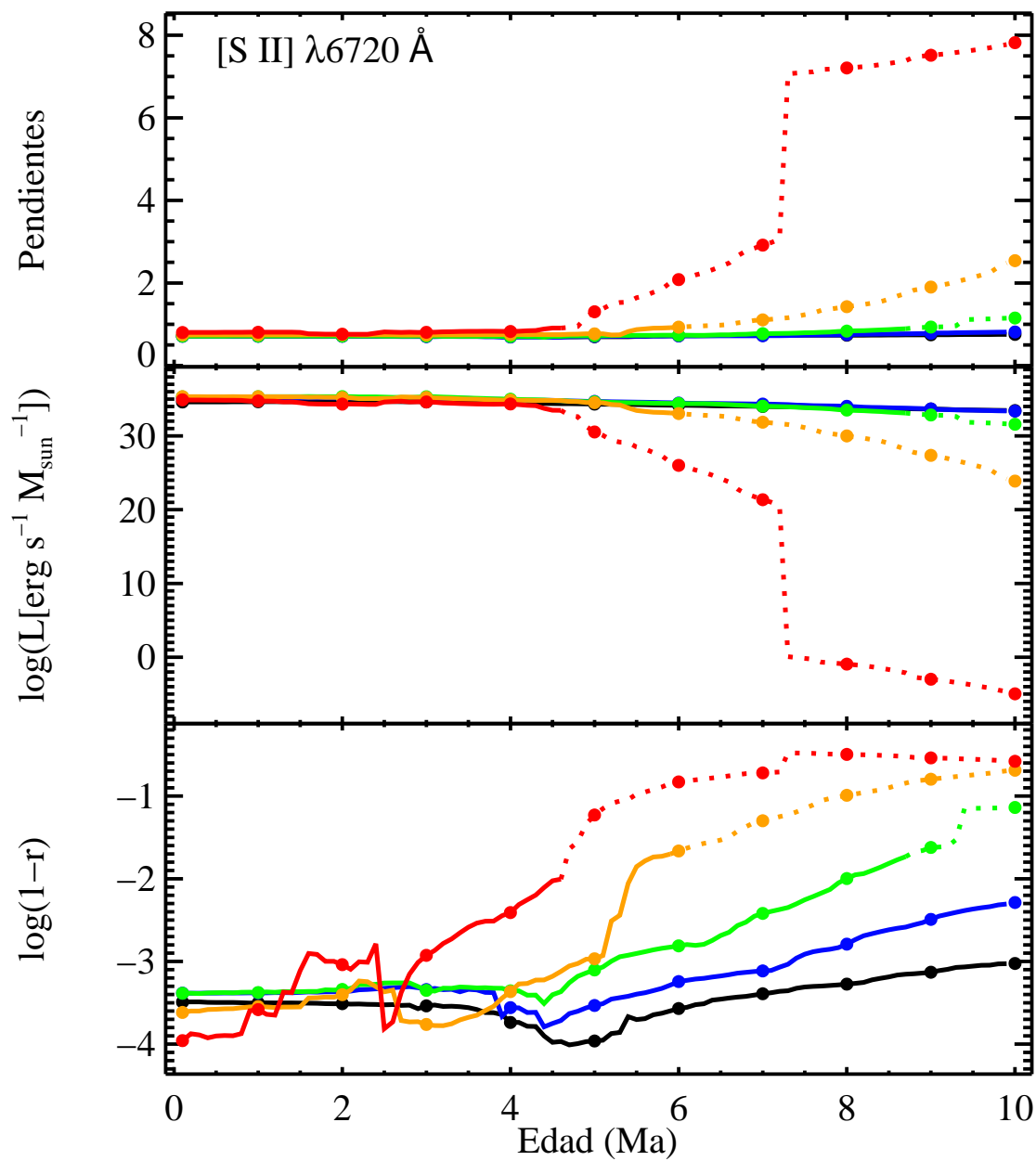
FIGURA A.20: Pendientes, \log L(1 M_{\odot}) y \log(1-r) para [S II] \lambda 6720 \text{ \AA} .
